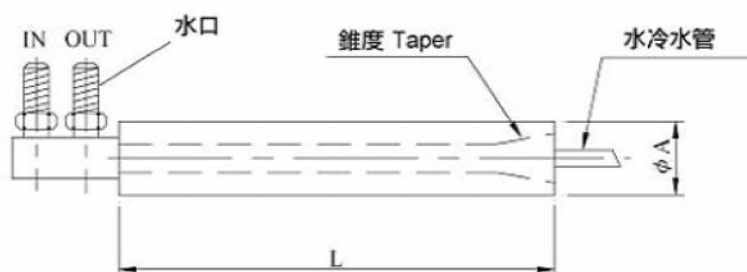
電極本體 Holder
